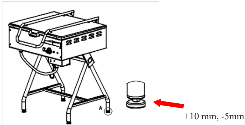
Bild 3. Ausnivellieren des Gerätes
